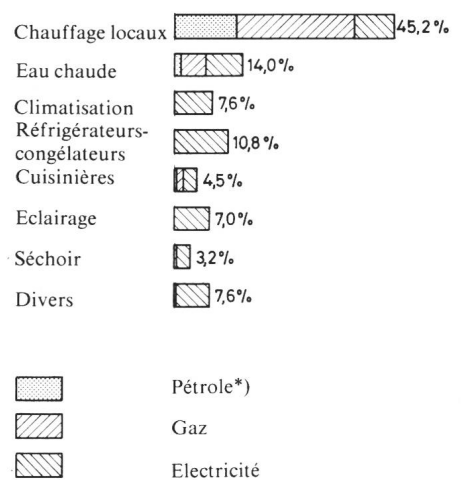
Fig. 1 Consommation approximative du secteur résidentiel en 1980 100% = 15,7 \cdot 10^{15} BTU = 16,6 EJ
