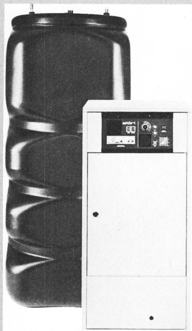
Elektro-Zentralspeicher mit Normkunststoffspeichern
