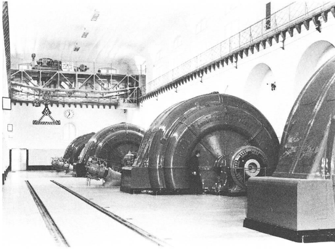
Fig. 8b Maschinensaal im SBB-Kraftwerk Ritom
