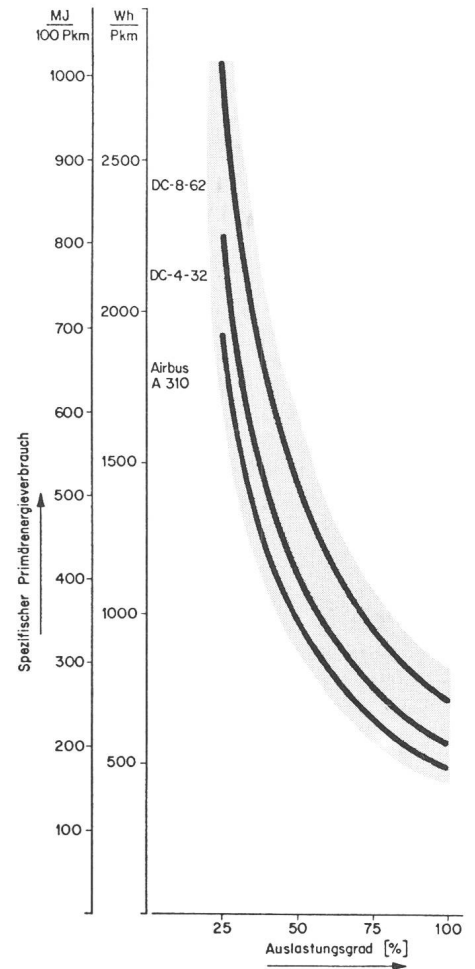
Fig. 5 Spezifischer Primärenergieverbrauch verschiedener Flugzeugtypen in Abhängigkeit der Auslastung auf der Strecke Zürich-Athen
