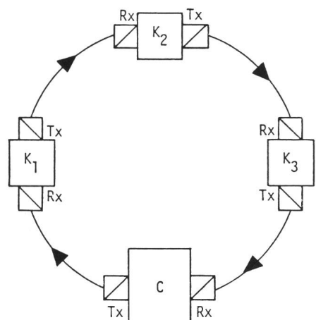
Fig. 1 Optisch-elektrisches (hybrides) LAN
