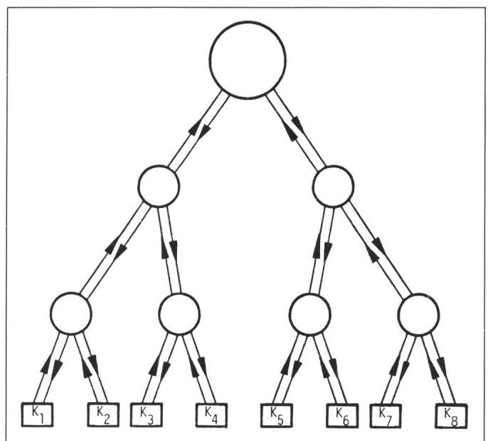
Fig. 8 Passives, aus 2x1-Kopplern aufgebautes FO-LAN in Baumtopologie
