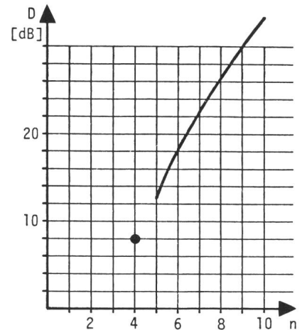
Fig. 7 Maximale Dämpfung zwischen zwei Anschlüssen eines FO-LAN mit Busstruktur in Funktion der Teilnehmerzahl
