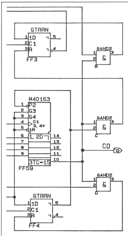
Fig. 6 Bildschirmansicht einer Schemaeingabe mit Symbol- und Signalbezeichnungen
