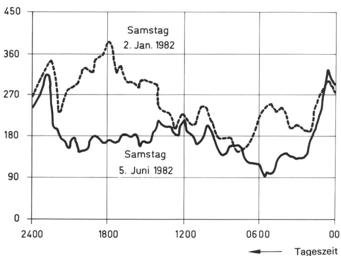
Belastung Trafo "Dorf" kW
