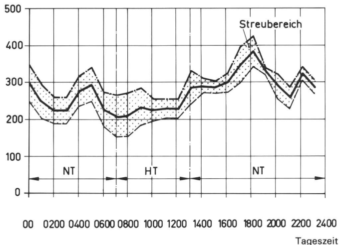
Fig. 5 Samstagsbelastung Trafo «Dorf» im Januar 1983: Die linke Figur zeigt die statistische Auswertung der Tagesganglinien (Mittelwert und Standardabweichung nach oben und unten). Die rechte Figur zeigt die an Samstagen gültigen Rundsteuerungszeiten
