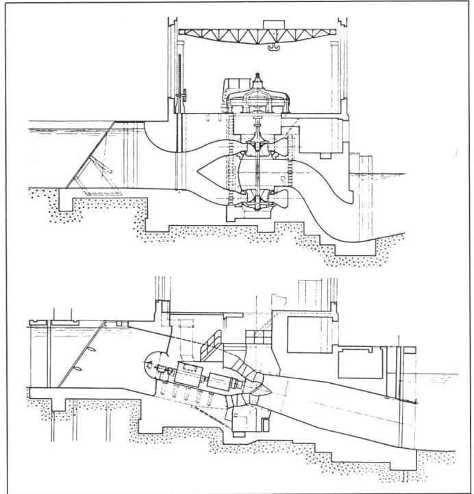
Fig. 1 Maschinenhausquer- schnitte des alten (oben) und des erneuerten und modernisierten (unten) Wasserkraftwerkes Au in Baden
