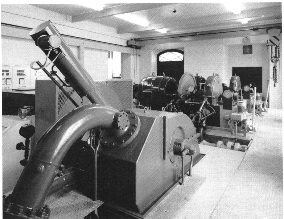
Fig. 2 Maschinensaal des erweiterten und modernisierten Wasserkraftwerkes Niederurnen
