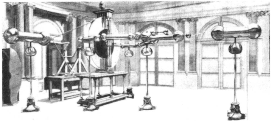
Fig. 1 Doppelscheiben-Elektisiermaschine nach Martin van Marum (1785)
