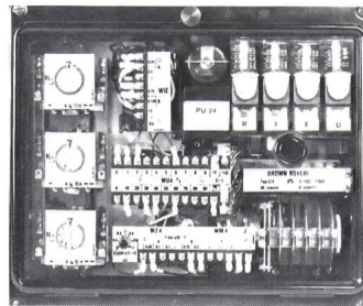
Distanzrelais Type LI 4/a BBC
