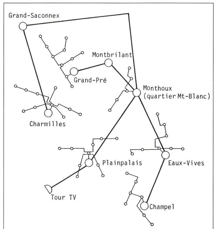
Fig. 2 Genève-Ville, Télé-réseau — Câbles à fibres optiques — Câbles coaxiaux dans canalisations PTT
