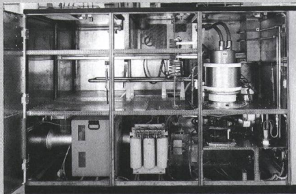
Geöffnete Hochfrequenz-Endstufe des ICRH-Verstärkers
