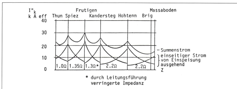
Figur 2 Subtransiente Kurzschlussströme und Impedanzen im Fahrleitungszug
