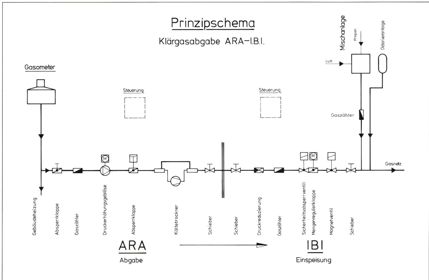
Figur 1 Prinzipschema der Klärgasabgabe ARA-IBI
