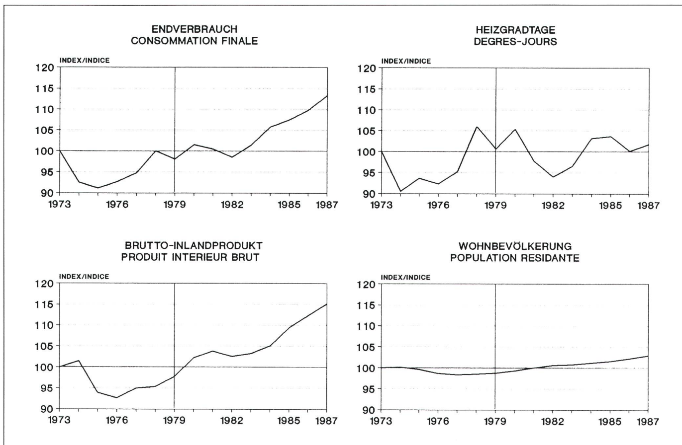
Fig. 1 Entwicklung des Endverbrauchs, der Heizgradtage, des realen Bruttoinlandproduktes und der Wohnbevölkerung im Vergleich Comparaison de l'évolution de la consommation finale d'énergie, des degrés-jours de chauffage, du produit intérieur brut réel et de la population résidente
