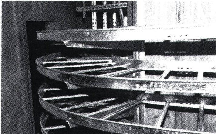
Kabelpitschen/Formstücke Breiten 200–600 mm, Randhöhe 60 mm ab Lager lieferbar
