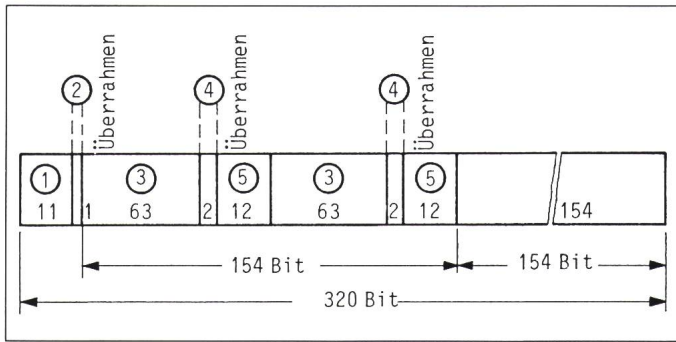
Figur 5 Hauptrahmen der Satellitenübertragung
