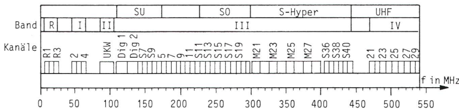
Figur 7 Vorschlag zur Neubelegung der Kabelkanäle S2-S41 unter Berücksichtigung des digitalen Rundfunks und der Einführung von Breitbandfernsehkanälen
