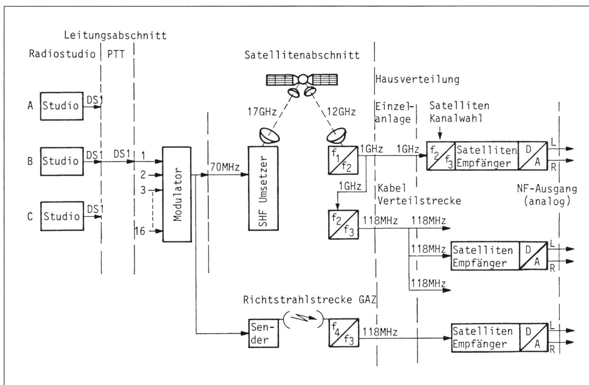
Figur 1 Übertragungsmöglichkeiten eines digitalen Radiosignals GAZ: Gemeinschaftsantennen-Zubringernetz der schweizerischen PTT
