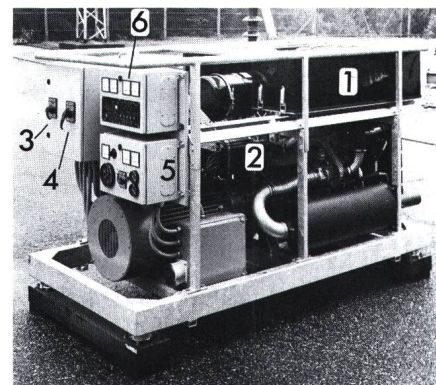
Figur 6 Ansicht des DAT-Generators
