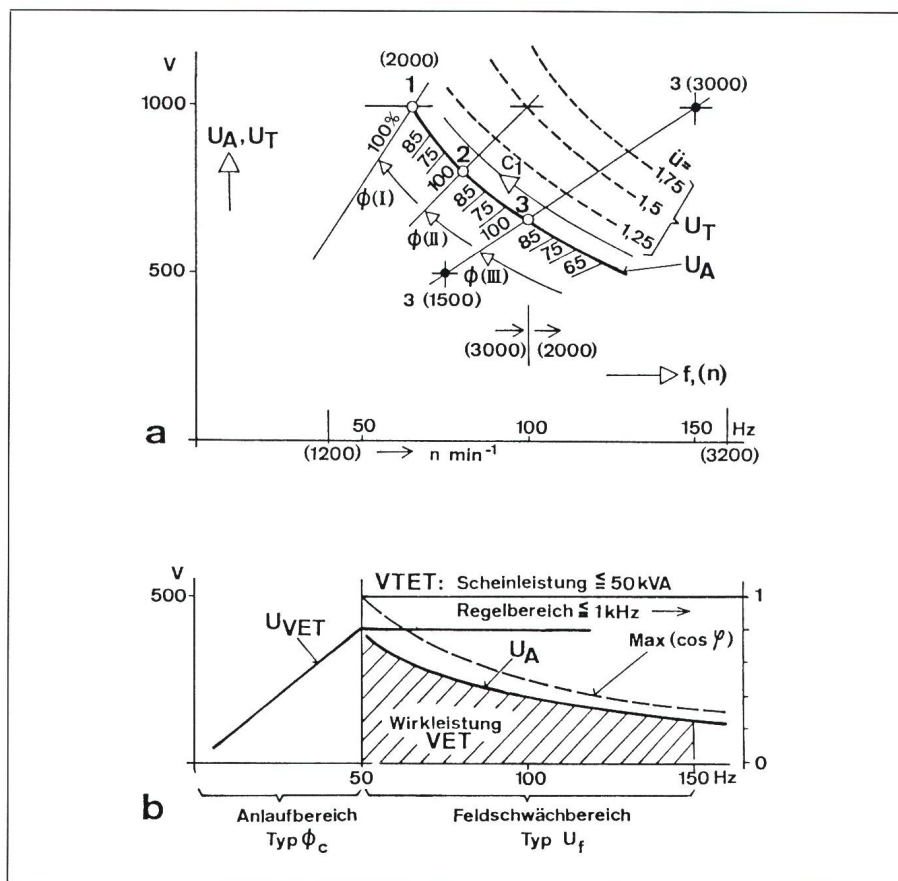
Figur 2 Spannungscharakteristiken U(f) , Resonanzlastanpassung der Stromquellen
