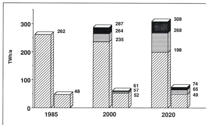
Figur 1 Entwicklung des Endenergie- und Stromverbrauchs in Baden-Württemberg (Referenzszenarien)
