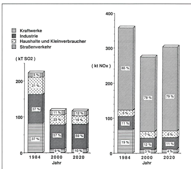
Figur 2 Entwicklung der SO 2 - und NO x -Emission nach Emittentengruppen (mittleres Referenzszenario)
