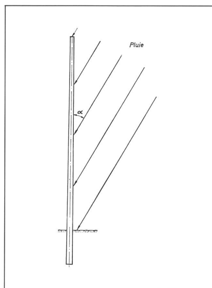
Figure 1 Accumulation d'eau au pied d'un poteau
