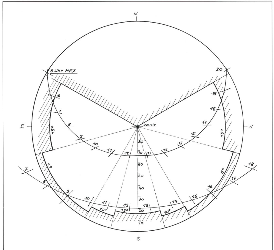
Figur 1 Idealhorizont für die Grobbeurteilung von Standorten. Darstellung in der Himmelskugel mit Angaben über tiefsten und höchsten Sonnenstand.
