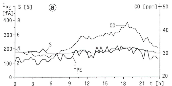
Figur 10 Tagesverlauf der CO- und der PAK-Konzentrationen sowie der Sichttrübung in Strassentunnel
