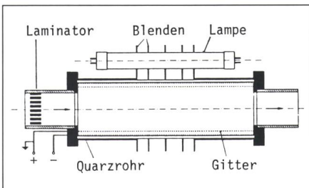
Figur 5 Aufbau der Photoemissionskammer
