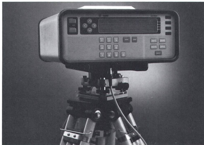
Bild 11 GPS-Empfänger für geodätische Anwendungen
