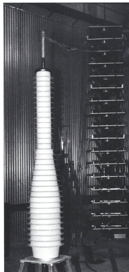
Bild 8 170 kV-Freiluftkabelendverschluss mit Silikonbeschirmung Produkt der Firma Dätwyler, Altdorf
