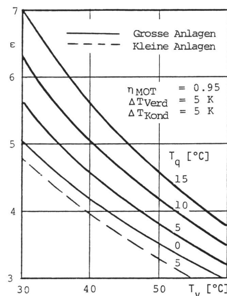
Bild 4 Leistungsziffern einstufiger Wärmepumpen
