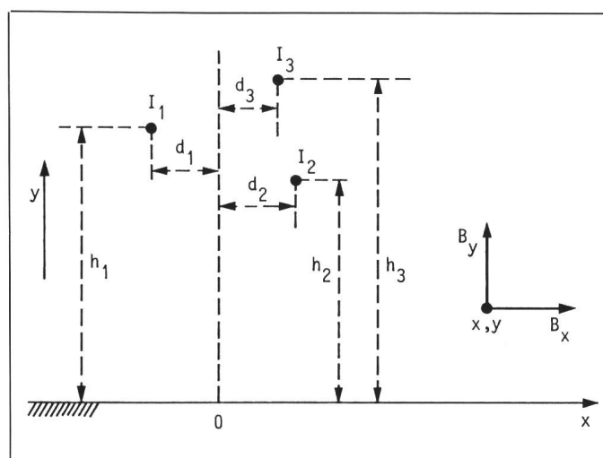
I_i courant de la phase i d_i, h_i coordonnées des conducteurs
