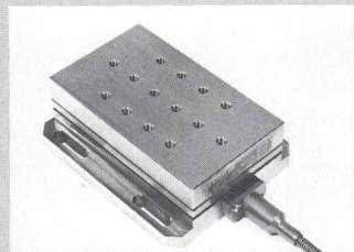
Piezoelektrisches Dreikomponenten-Dynamometer 9257B
