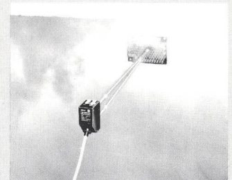
Lichtschranken für Flüssigkeiten
