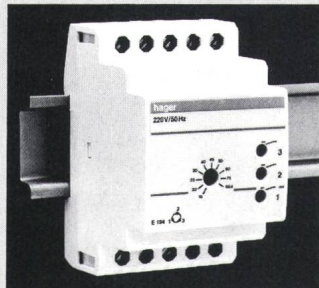
Délesteur 3 voies tournantes
