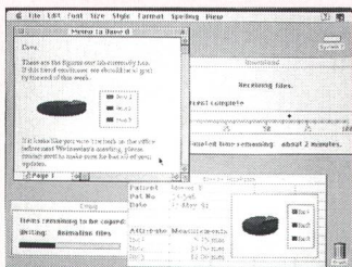
Benutzeroberfläche System 7
