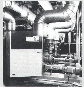
Pulsumrichter
