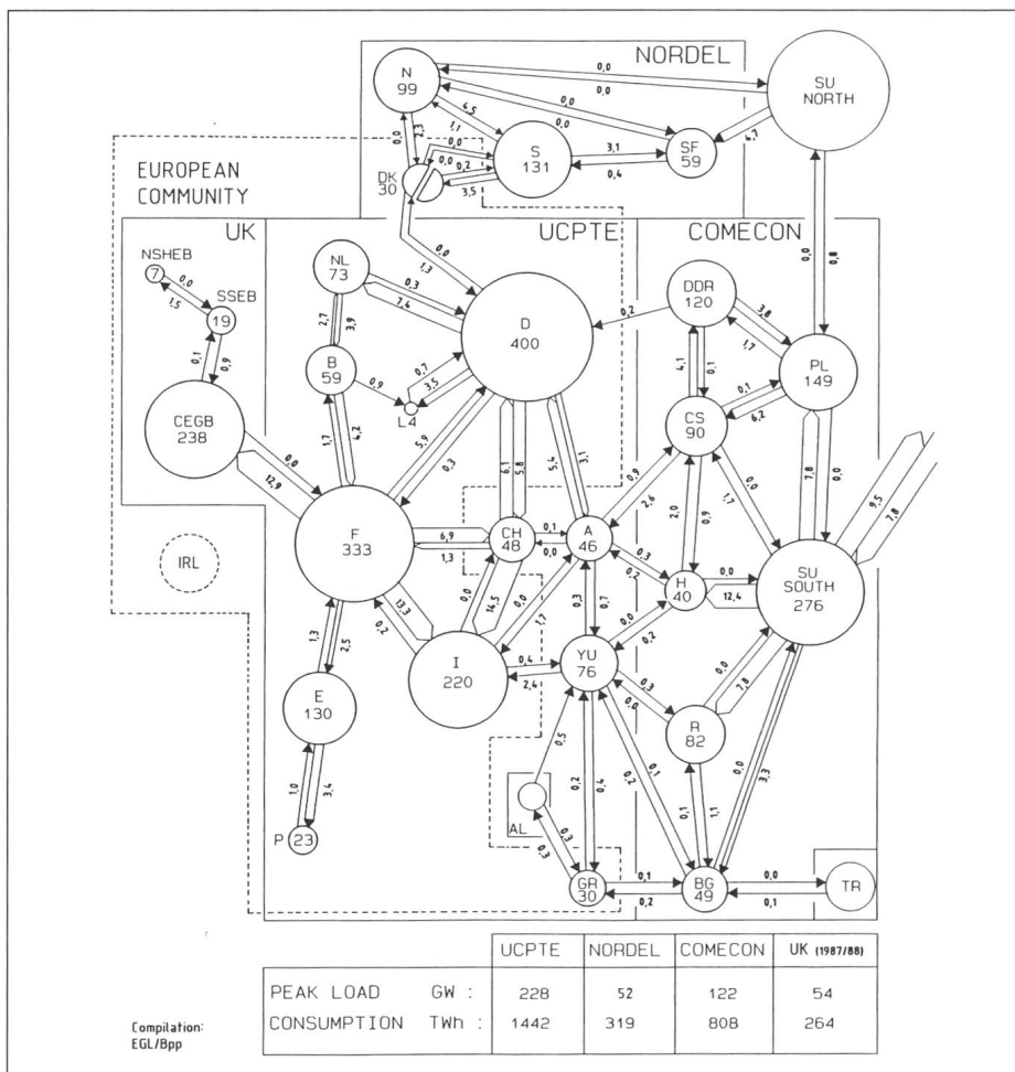
Bild 2 Elektrizitätsverbrauch und Stromtausch der europäischen Länder im Jahr 1988 (in TWh)
