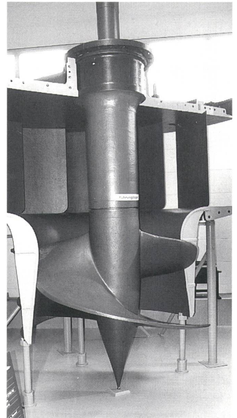
Schraubenturbine (Schnelläufer) aus dem Jahr 1924 aus dem Kraftwerk Matte des Elektrizitätswerkes Bern
