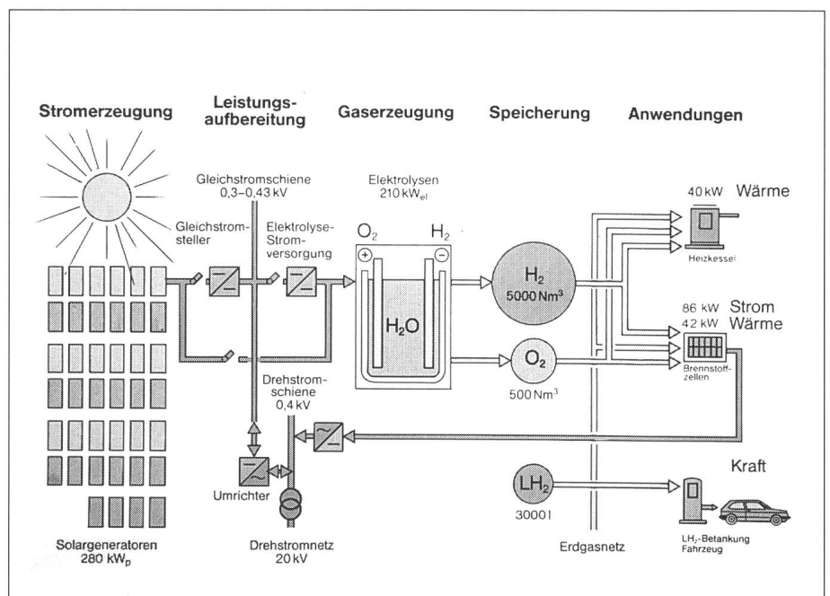
Bild 8 Die Schritte von Wasserstoffgewinnung und -anwendung, die in Neunburg erprobt werden: Die Solarzellen liefern Gleichstrom für die Wasser-Elektrolyse (der Stromüberschuss wird als Drehstrom ins Netz gespeist); Wasserstoff und ein Teil des Sauerstoffs werden gespeichert und dann in Heizkesseln und Brennstoffzellen in Wärme- und Elektroenergie umgesetzt. Flüssigwasserstoff zum Versuchsbetrieb von Wasserstoffautos kommt von auswärts Grafik SWB
