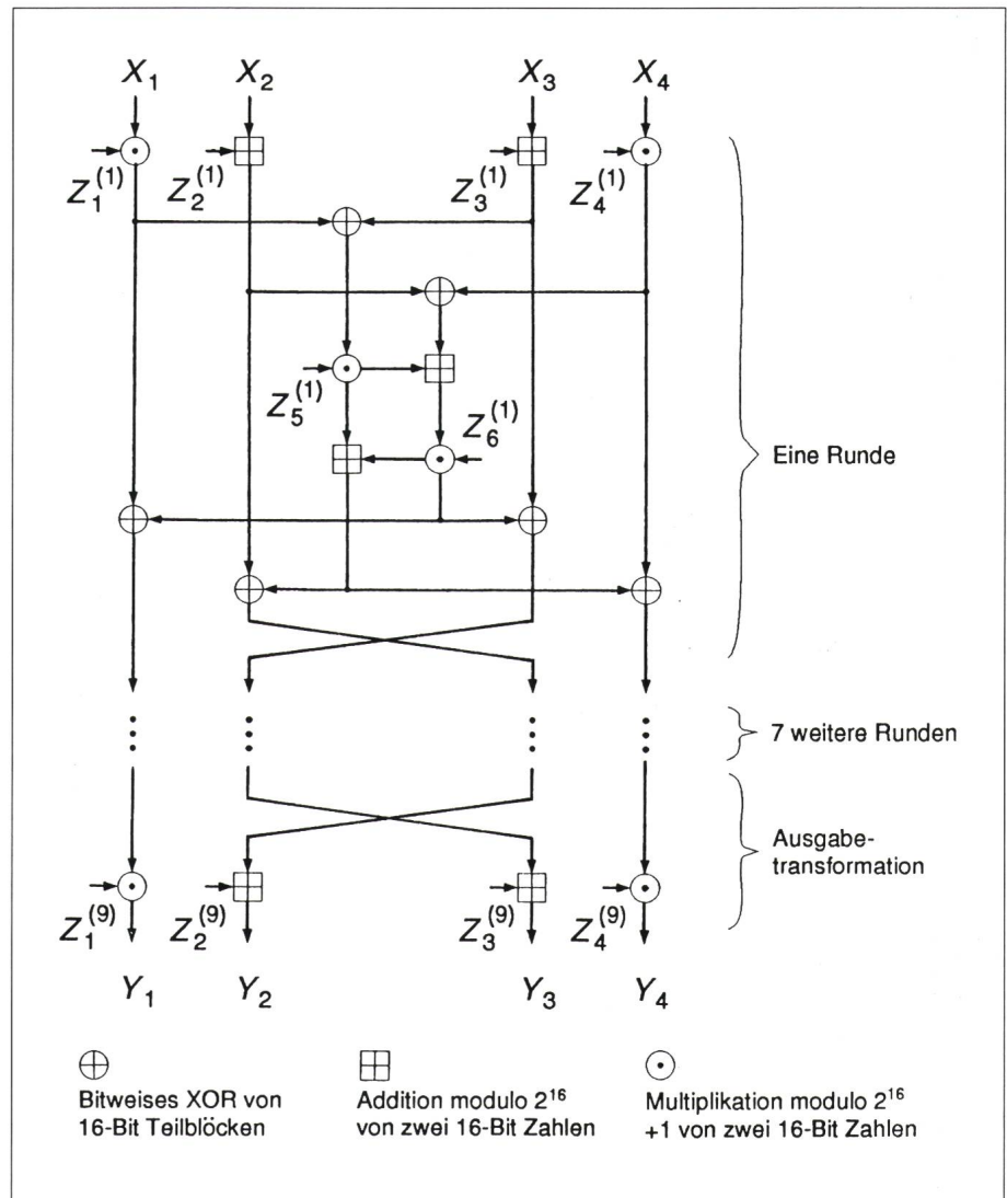
Bild 1 Datenfluss des Idea-Algorithmus
