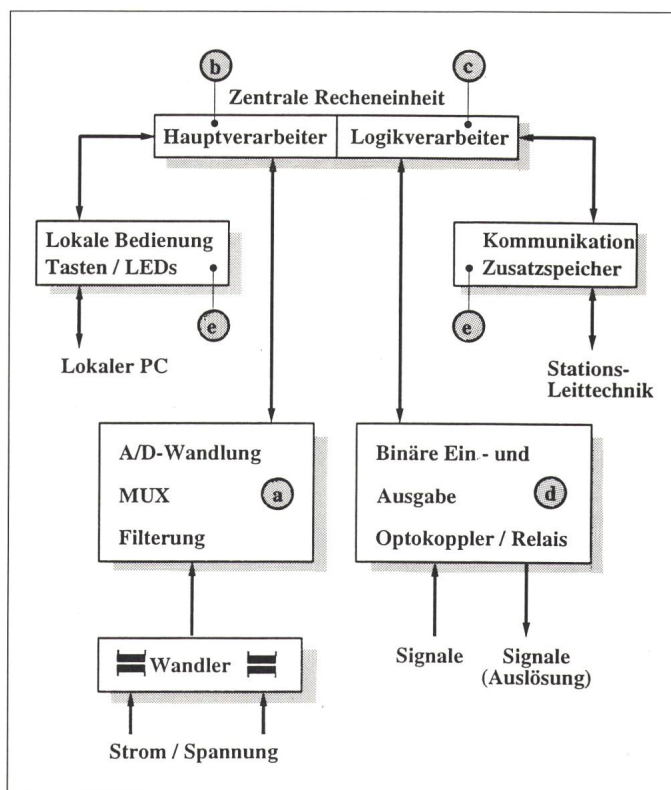
Bild 1 Hardware-Struktur
