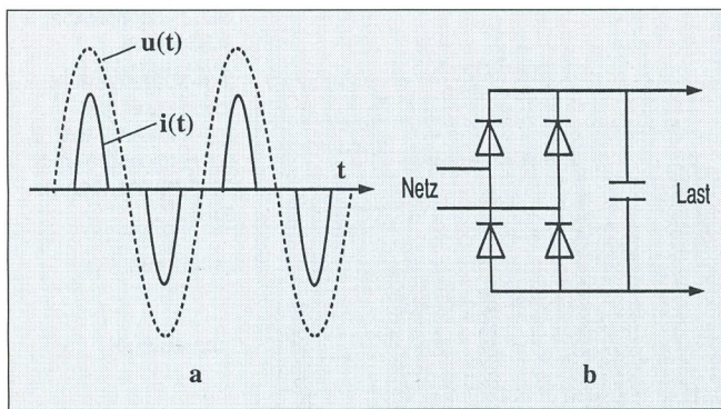
Bild 4 Kapazitive Glättung (einphasig) a Verlauf von Netzspannung u(t) und Netzstrom i(t) b Prinzipschema
