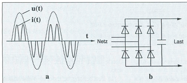
Bild 5 Kapazitive Glättung (dreiphasig) a Verlauf von Netzspannung u(t) und Netzstrom i(t) b Prinzipschema
