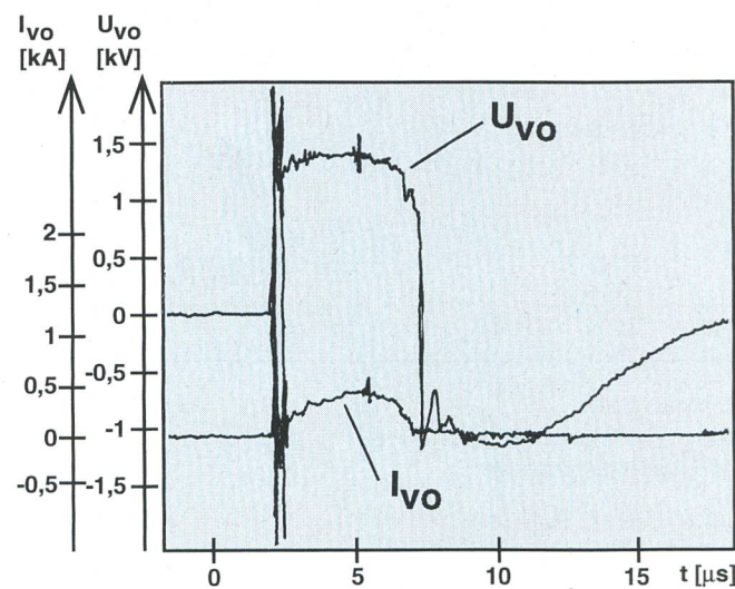
Bild 17 Strom und Spannung am wechselrichterseitigen Überspannungsableiter Strom I_{vo} und Spannung U_{vo} am Überspannungsableiter nach der abgeschirmten Leitung zum DC-Verbraucher (rechte Seite in Bild 15), unter den gleichen Bedingungen wie in Bild 16 [6]
