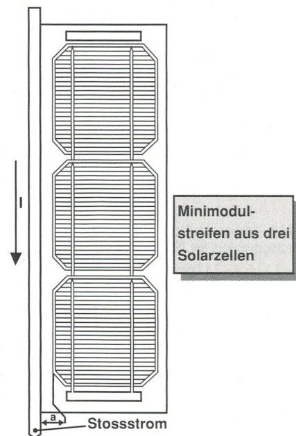
Bild 7 Testanordnung
