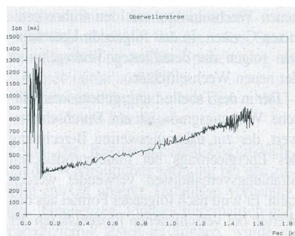
Bild 8 Effektivwert des Oberschwingungsstromes beim Top Class 1500 in Funktion der Ausgangsleistung
