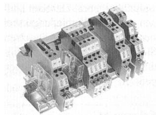
Dreistock-Installationsklemme
