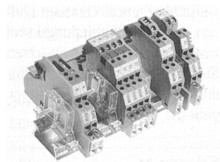
Dreistock-Installationsklemme
