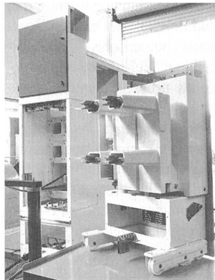
Vakuu-LS 24 kV, 1250 A mit Motorantrieb
