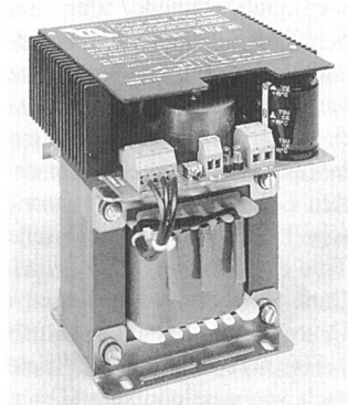
Fernsteuerbares Schaltnetzteil
