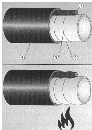
Aufbau des Kabels: 1 = Glasfaserkabel 2 = wachsgefüllter Schlauch 3 = Aramid-Faser 4 = Kunststoffmantel
