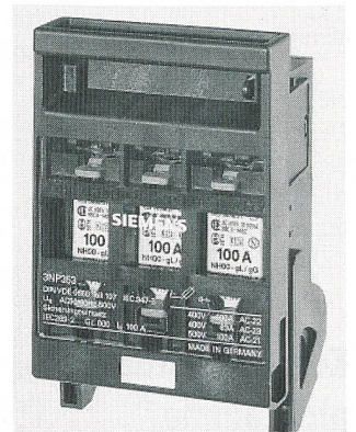
Sicherungs-Lasttrennschalter 3NP35
