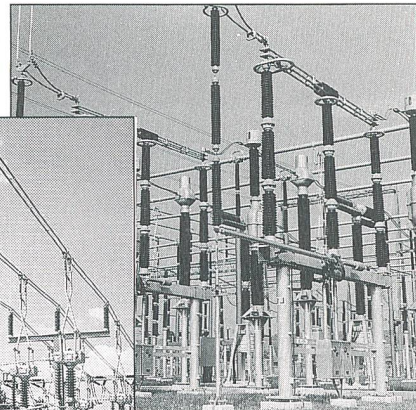
Drehtrenner: 170-420 kV
