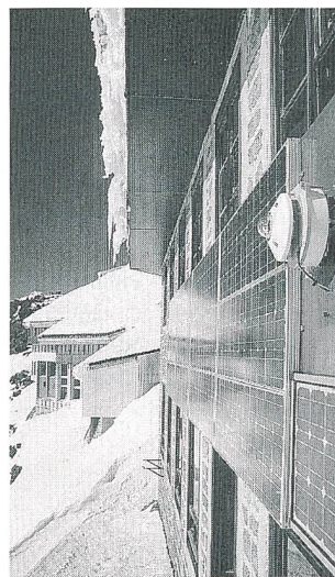
Höchstgelegene netzgekoppelte Photovoltaik-Forschungsanlage auf dem Jungfraujoch
