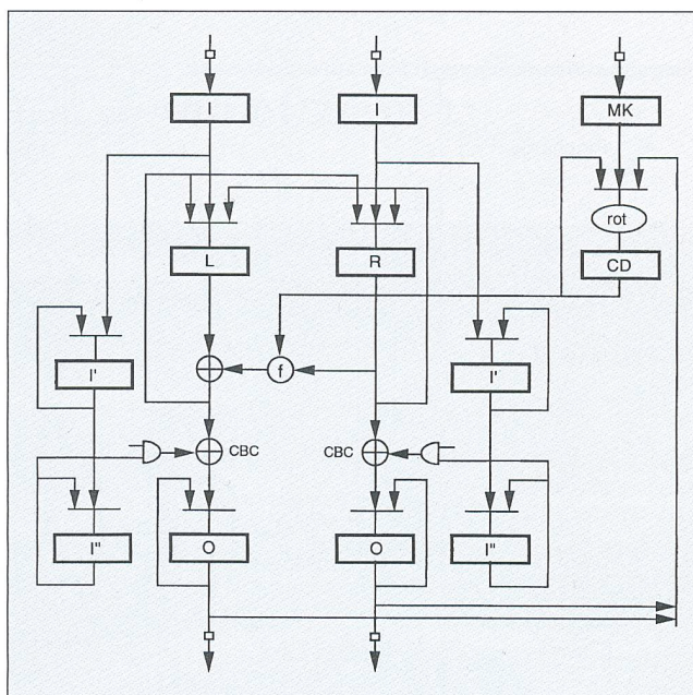
Bild 6 Dechiffrieren
