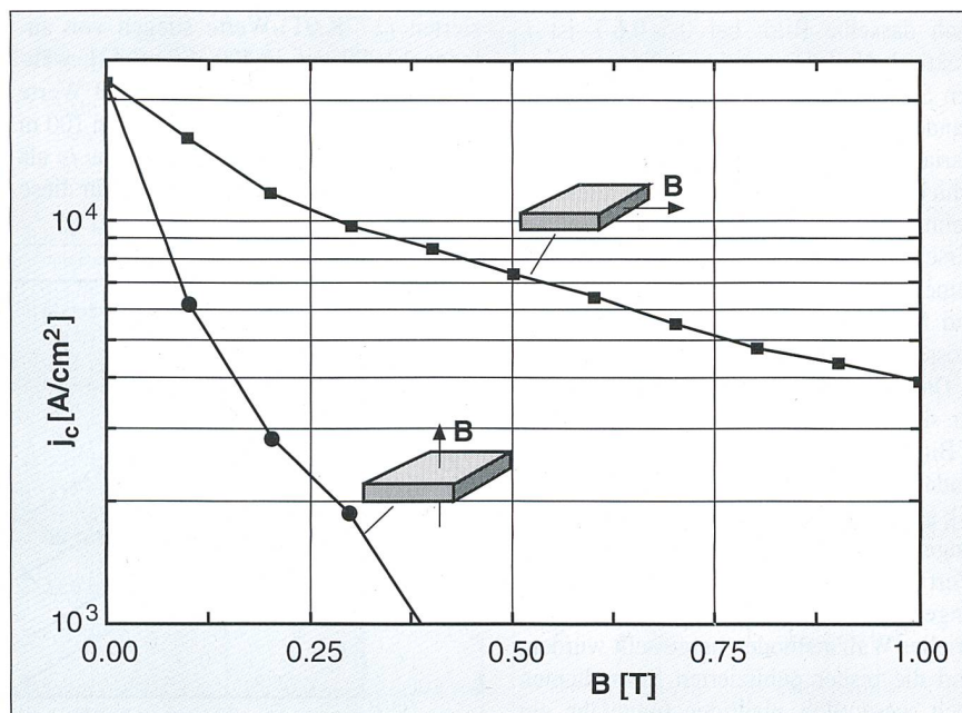
Bild 7 Kritische Stromdichte eines langen, gewalzten Bi(2223)-Bandes
