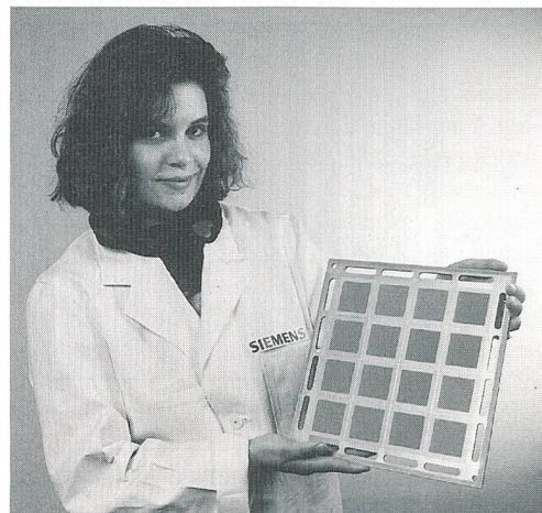
Bipolare Platte mit Brennstoffzellen
