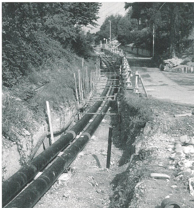
Mit Wärmetransportleitungen wird die Abwärme zu den Wärmebezüglern der Refuna transportiert
