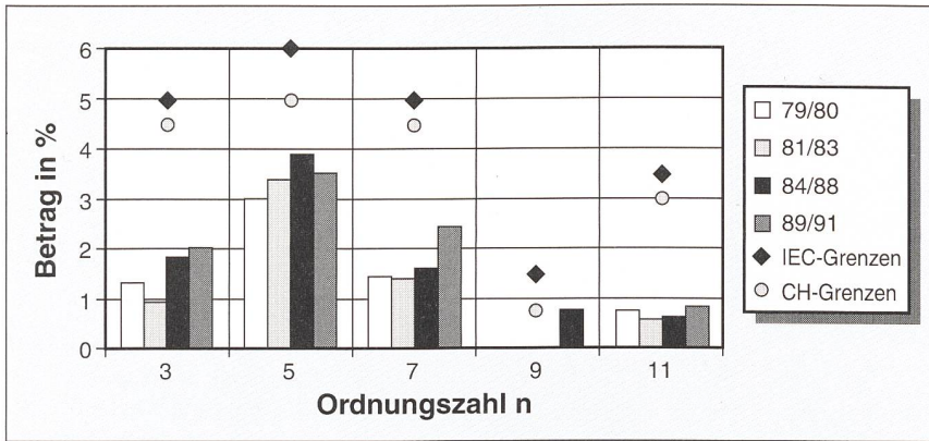
Bild 5 Spannungsoberschwingungen im Schweizer Niederspannungsnetz Entwicklung der Spannungsoberschwingungen über die Jahre (95%-Auftrittswahrscheinlichkeit), verglichen mit den Kompatibilitätspegeln nach IEC und SEV 3600.
