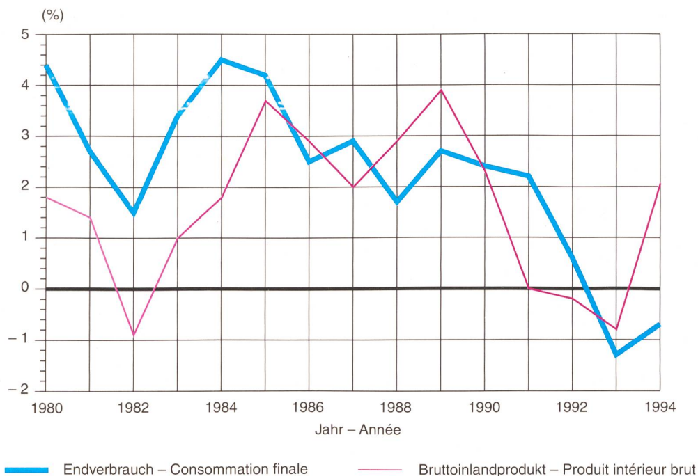
Fig. 4 Veränderungsraten Stromverbrauch – Bruttoinlandprodukt real 1
