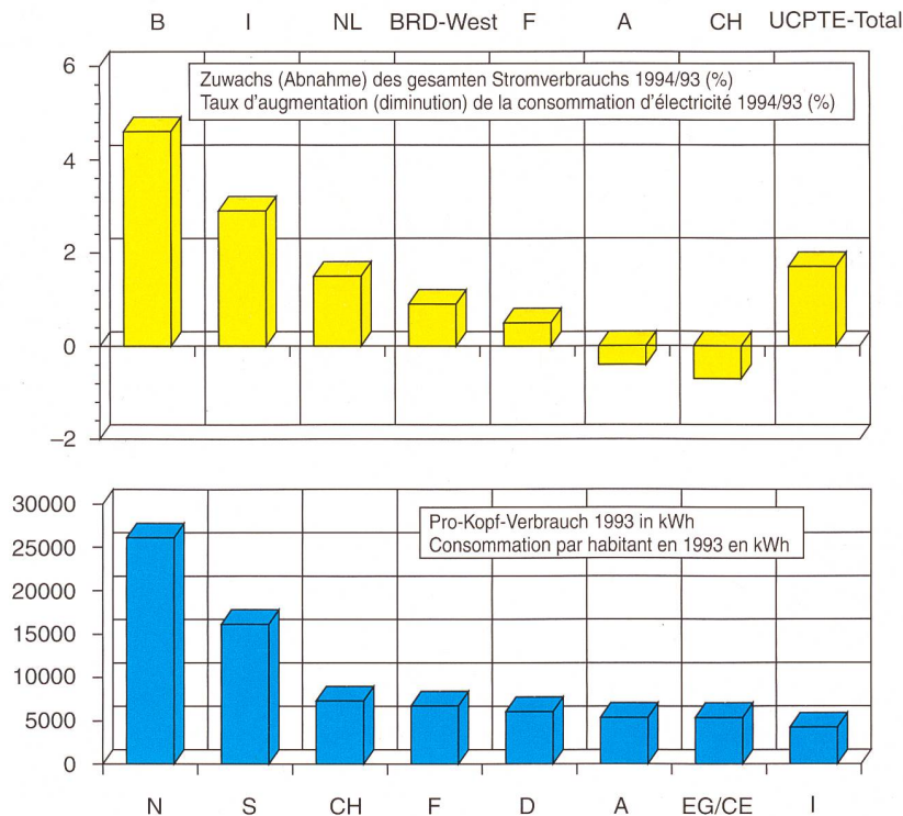
Fig. 6 Consommation de divers pays
