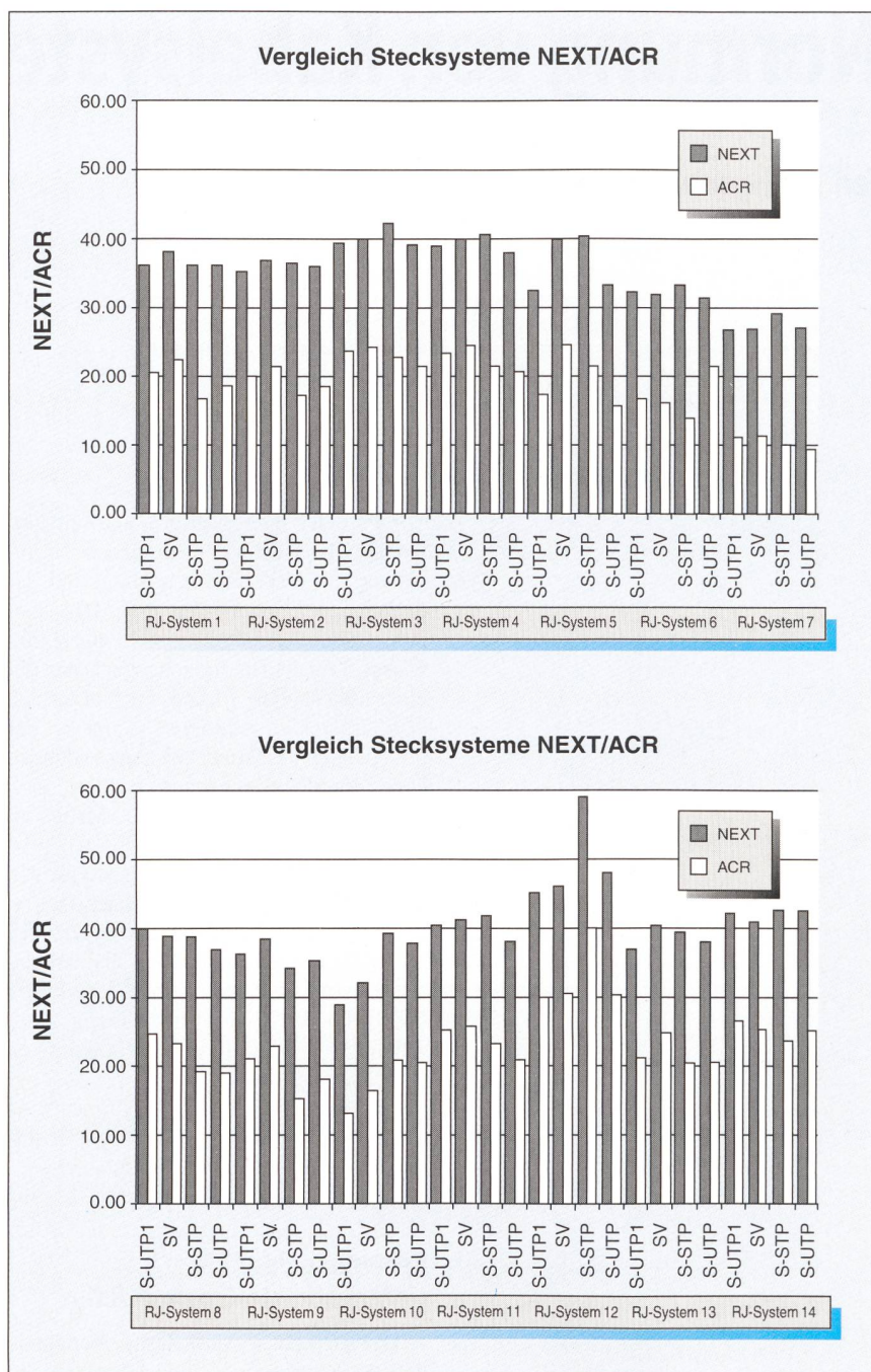
Bild 1 Vergleich Stecksysteme NEXT/ACR
