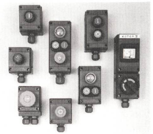
Befehlsgerätereihe in explosionsgeschützter Ausführung
